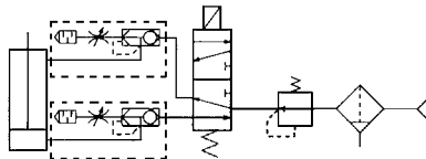
Cilindar sa ASV ventilom
